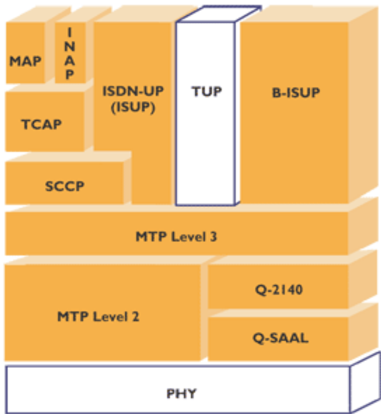
SS7
