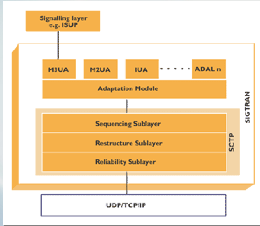
SIGTRAN
